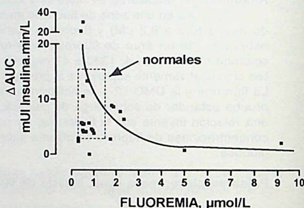
Fig. 1.— Relación entre el Área Bajo la Curva de Insulinemia durante una prueba estándar de tolerancia a la glucosa y la fluoremia de 26 sujetos residentes y ex-residentes de una zona de fluorosis endémica cercana a Bahía Blanca. El intervalo de confianza del 95% de los valores normales de las dos variables define el área rectangular marcada con línea de puntos.
