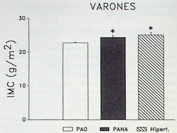
Fig. 3.— Barras que muestran el IMC en los tres grupos estudiados. Los grupos PANA e Hipertensos tuvieron IMC significativamente más elevados que el grupo PAO (P<0,05). No difirieron significativamente entre sí los grupos PANA e Hipert.
