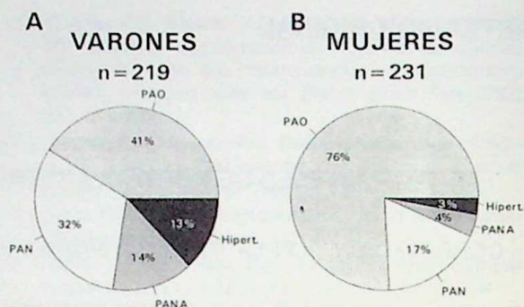
Fig. 1.— Muestra la prevalencia en varones y mujeres de las diferentes categorías según el Joint National Committee V. PAO: Presión Arterial Óptima; Hipert.: Hipertensos; PANA: Presión Arterial Normal Alta y PAN: Presión Arterial Normal. Note que PANA, PAN y PAO tienen presiones arteriales normales. La prevalencia de hipertensión en este grupo etáreo fue de 13% en varones, 3% en mujeres y 8% total.
