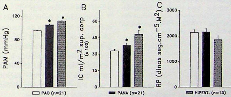
Fig. 5.— Muestra los hallazgos hemodinámicos en tres grupos de varones, PAO: presión arterial óptima, Hipert: Hipertensos y PANA: Presión Arterial Normal Alta. En A PAM, en B Índice Cardíaco y en C Resistencia Periférica normalizada por Superficie Corporal. La PAM y los IC de los grupos PANA e Hipert. fueron estadísticamente más elevados que en los del grupo PAO. El IC de los PANA fue diferente al de los Hipert.
