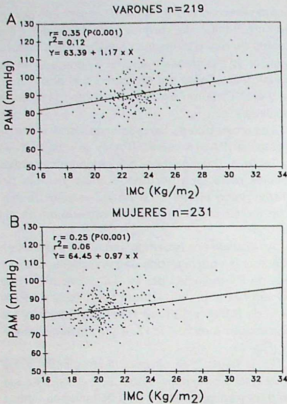
Fig. 2.— Muestra la correlación entre IMC y PAM en varones (panel A) y mujeres (panel B). Ambas correlaciones fueron estadísticamente significativas. La PAM incrementa en los varones 1,17 mmHg por cambio de 1Kg/m 2 de IMC y 0,97 de mmHG en las mujeres.
