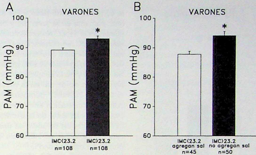
Fig. 4.— Muestra en el panel A los niveles de PAM en varones con IMC menor y mayor que la mediana y en el panel B se comparan los PAM de aquéllos con menor IMC que agregan sal con los PAM de las de mayor índice de masa corporal que no agregan sal en la mesa. El agregado de sal no corrigió las diferencias de la PA.
