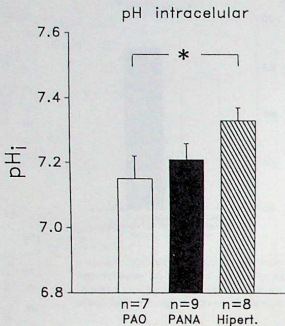
Fig. 6.— Muestra los valores de pHi en plaquetas de los tres grupos estudiados. Sólo el grupo hipertenso mostró aumentos estadísticamente significativos del pHi respecto a los grupos PAO y PANA los cuales no difirieron significativamente entre sí.
